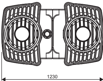
(DRAINBOX 600)
