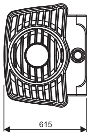
(DRAINBOX 300)
