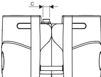
(DRAINBOX 600)
